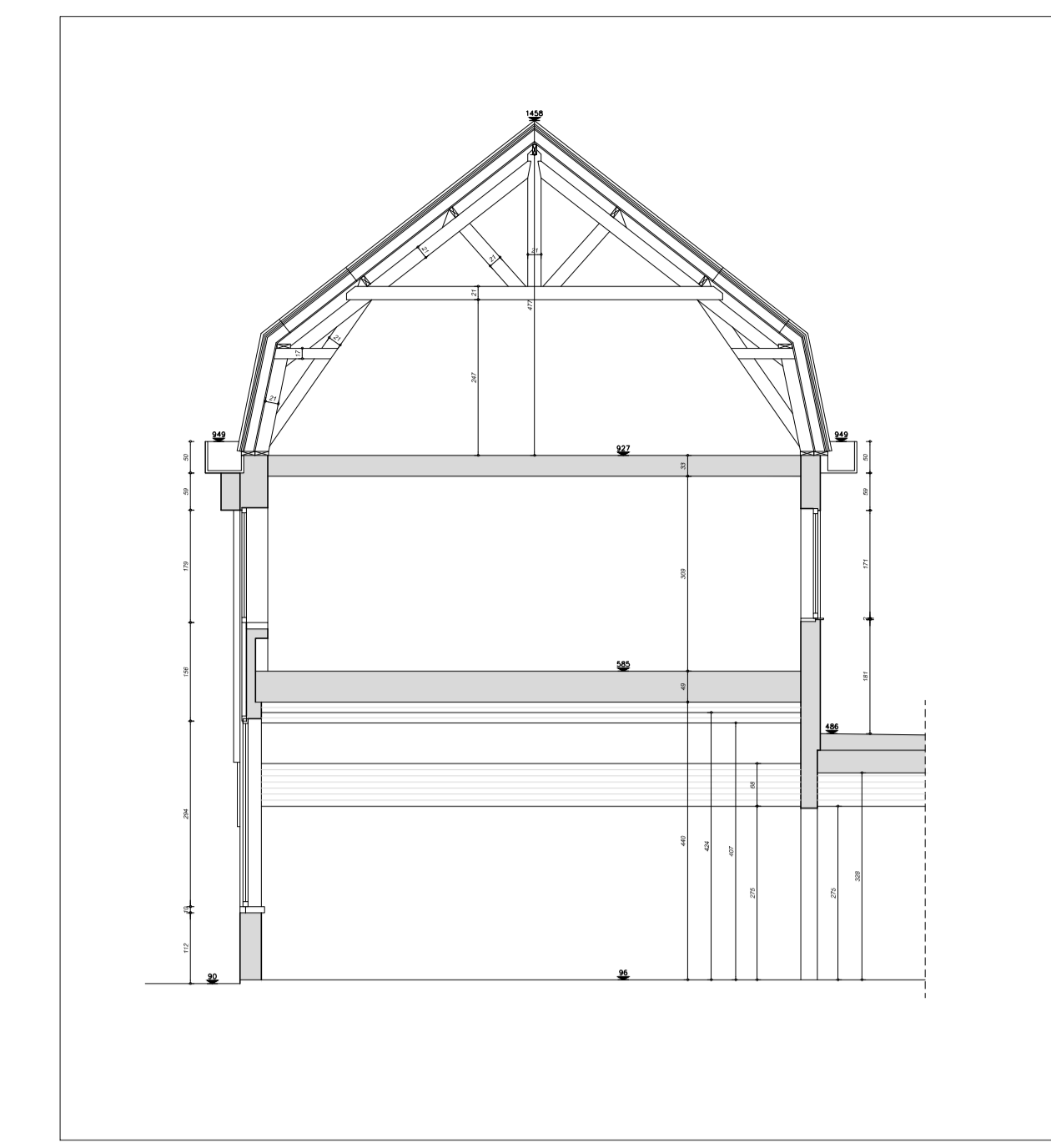
snede BB
