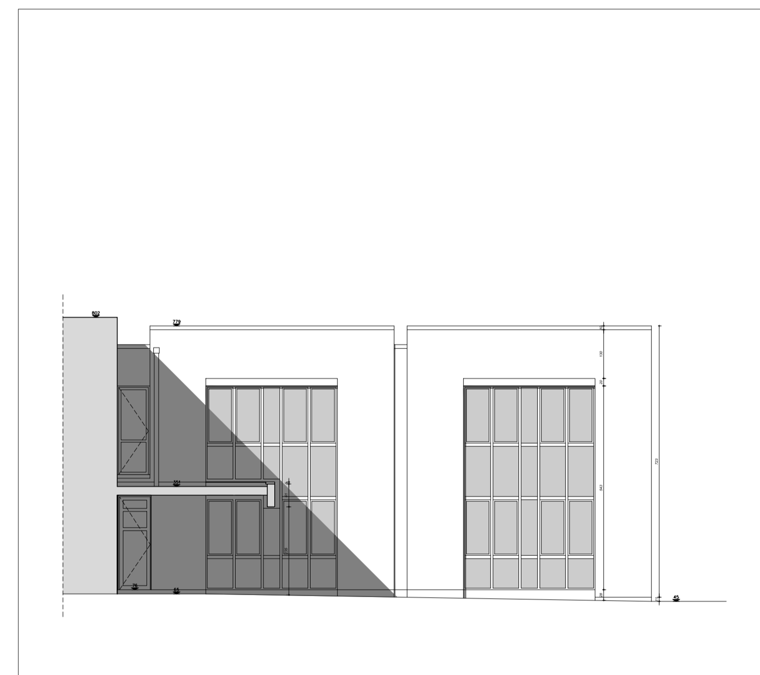
oostgevel middenbouw
