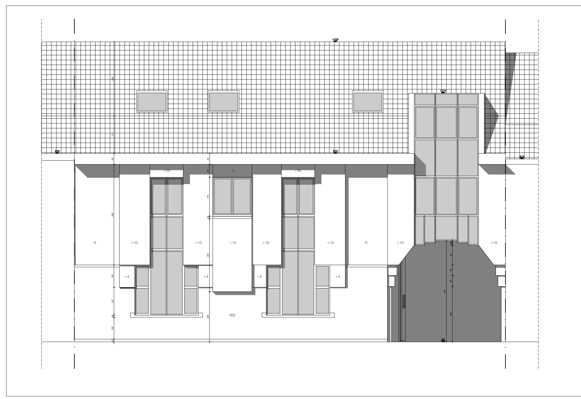
voorgevel veldstraat
