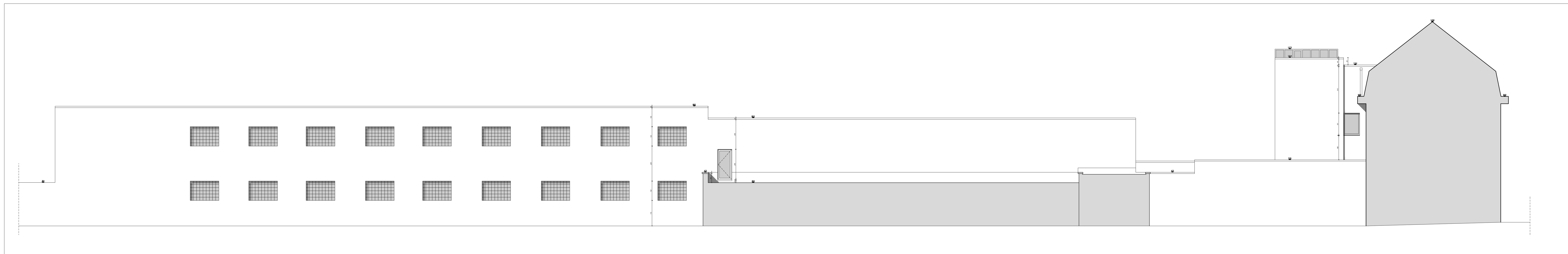
noordgevel middenbouw
