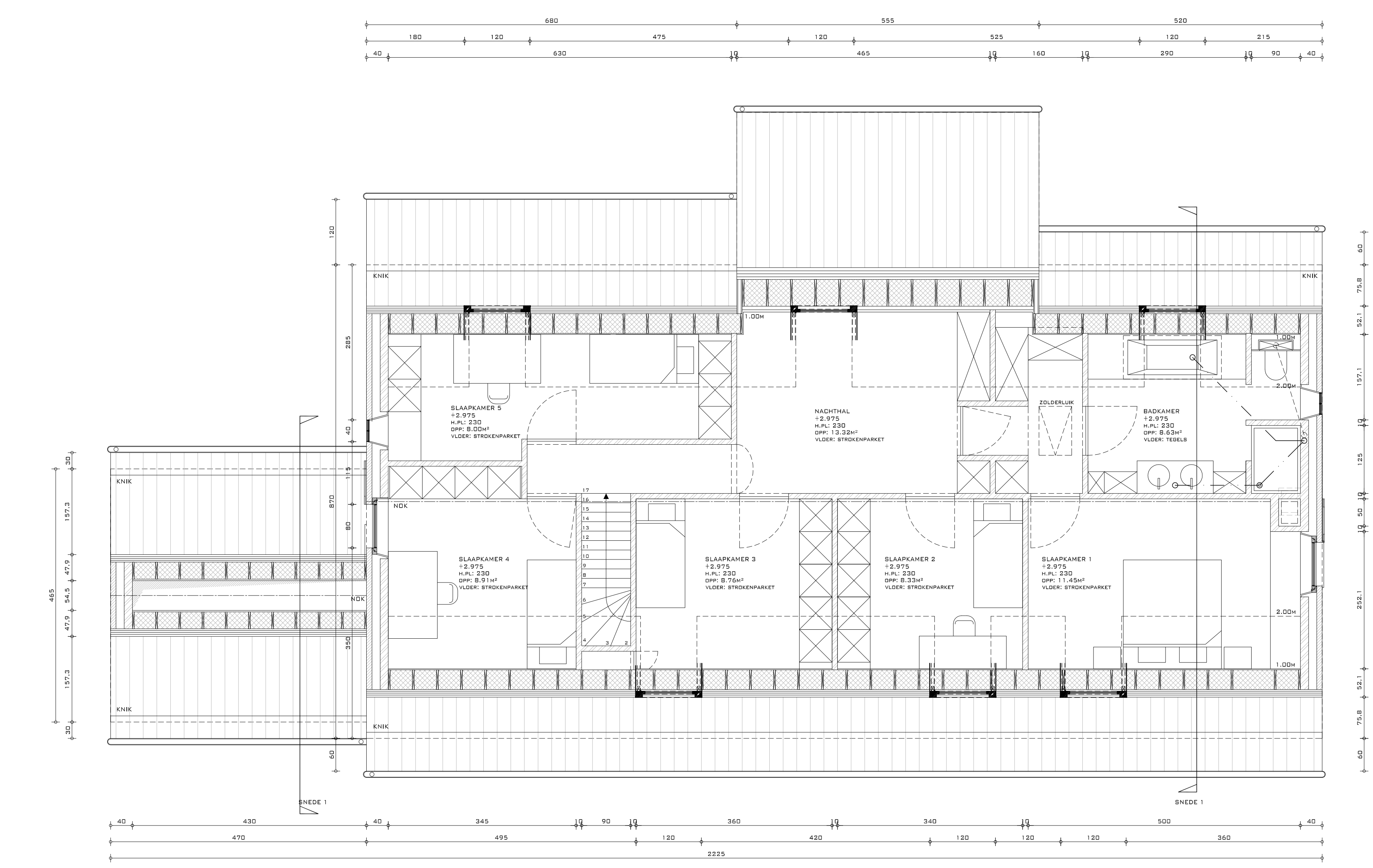
VERDIEPING
