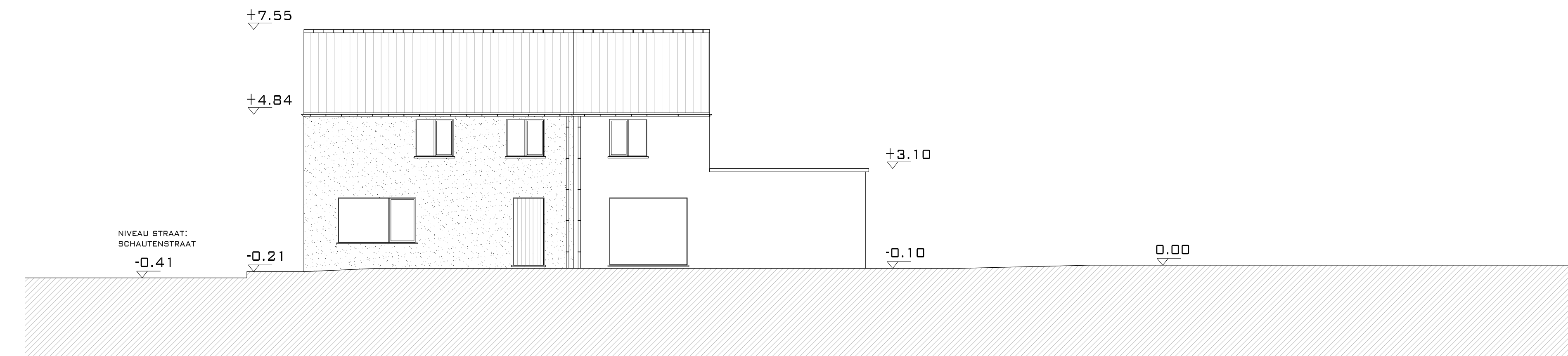
TERREINPROEFIEL NIEUWE TOESTAND - 1/100
