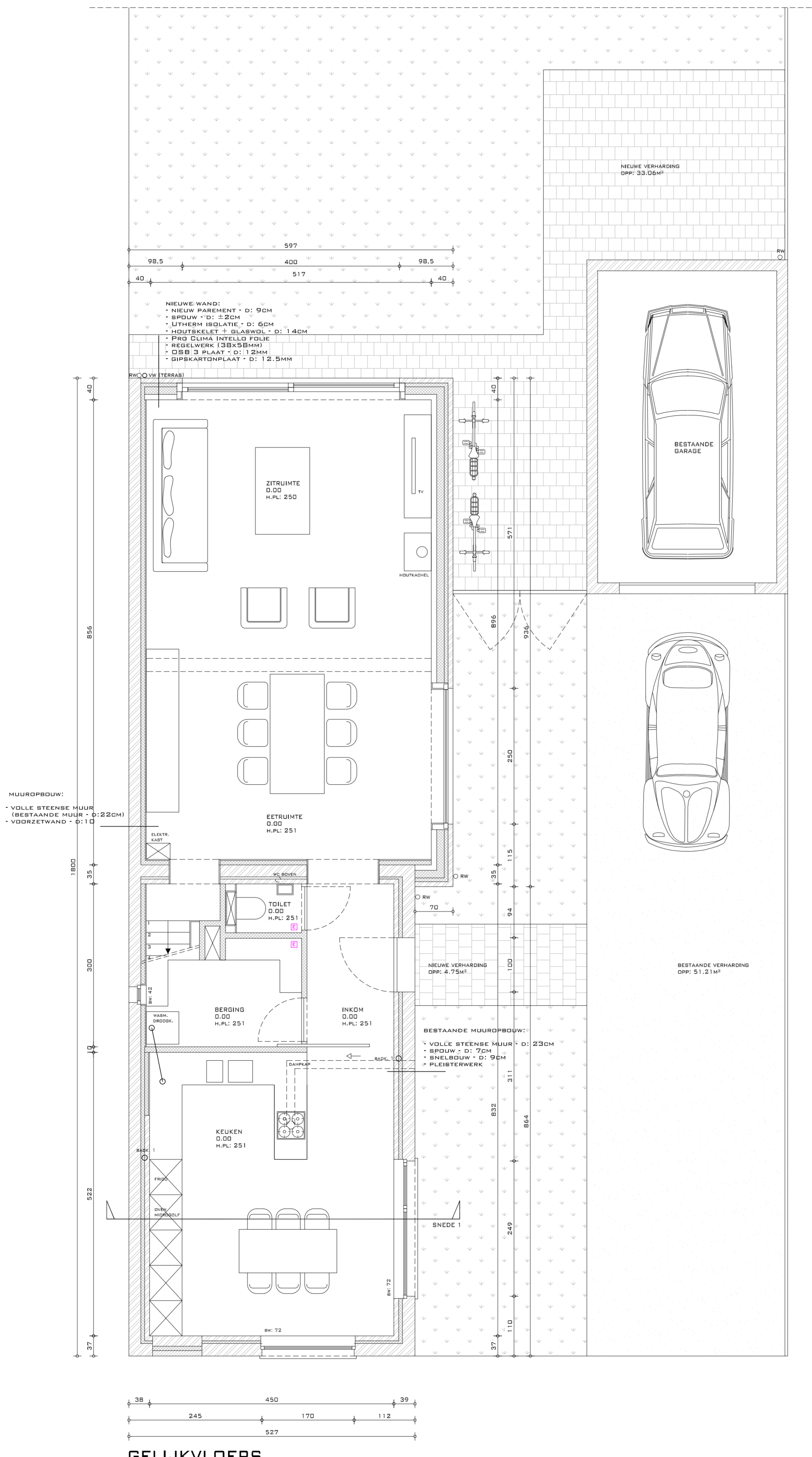
BELIJKVLOERS
