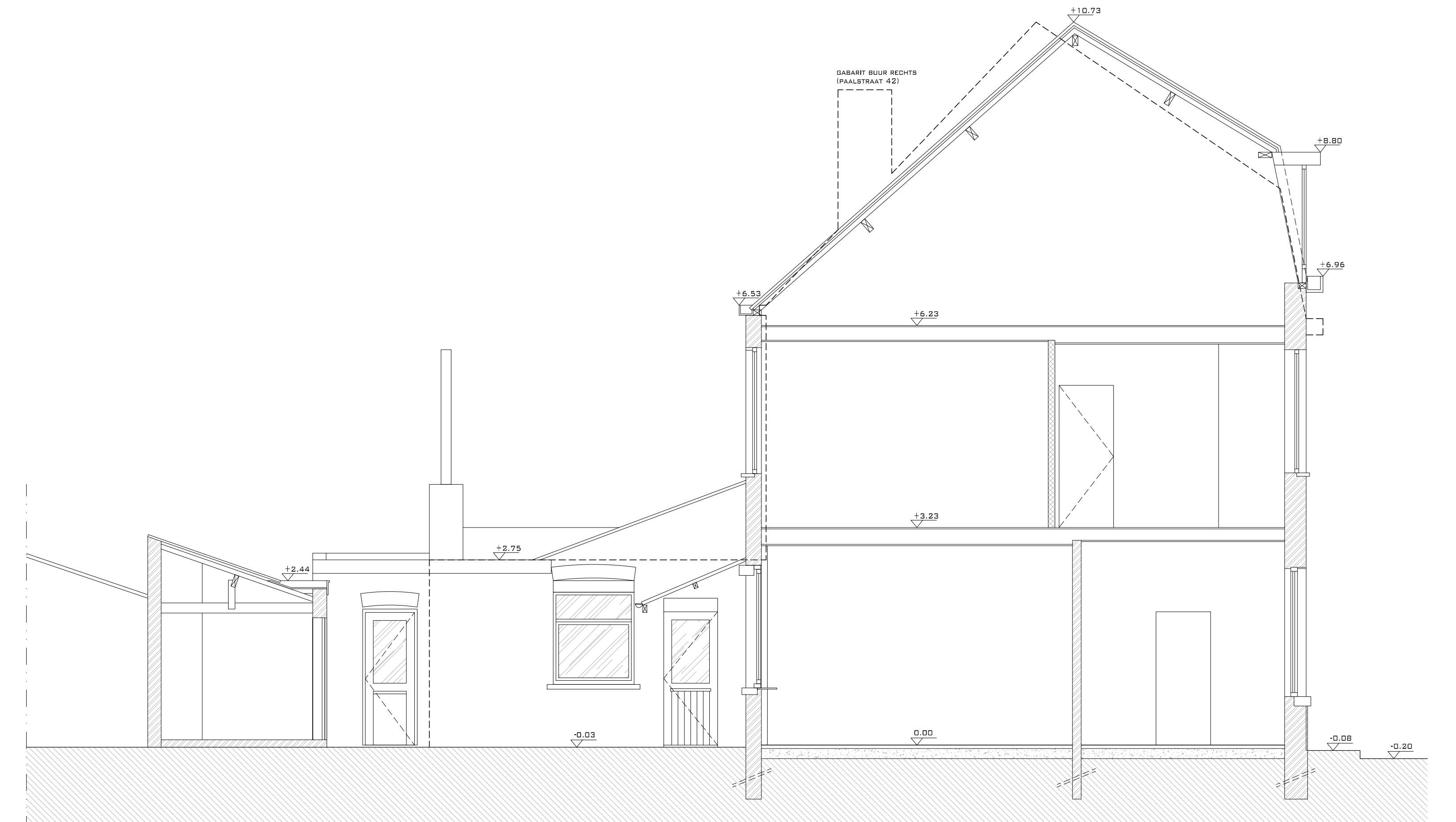
SNEDE 1 / ZIJGEVEL KEUKEN (+ GABARIT BUUR RECHTS)
