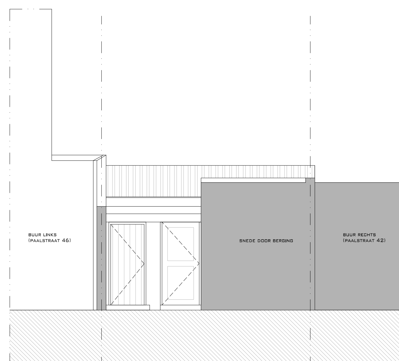
GEVEL WASPLAATS
