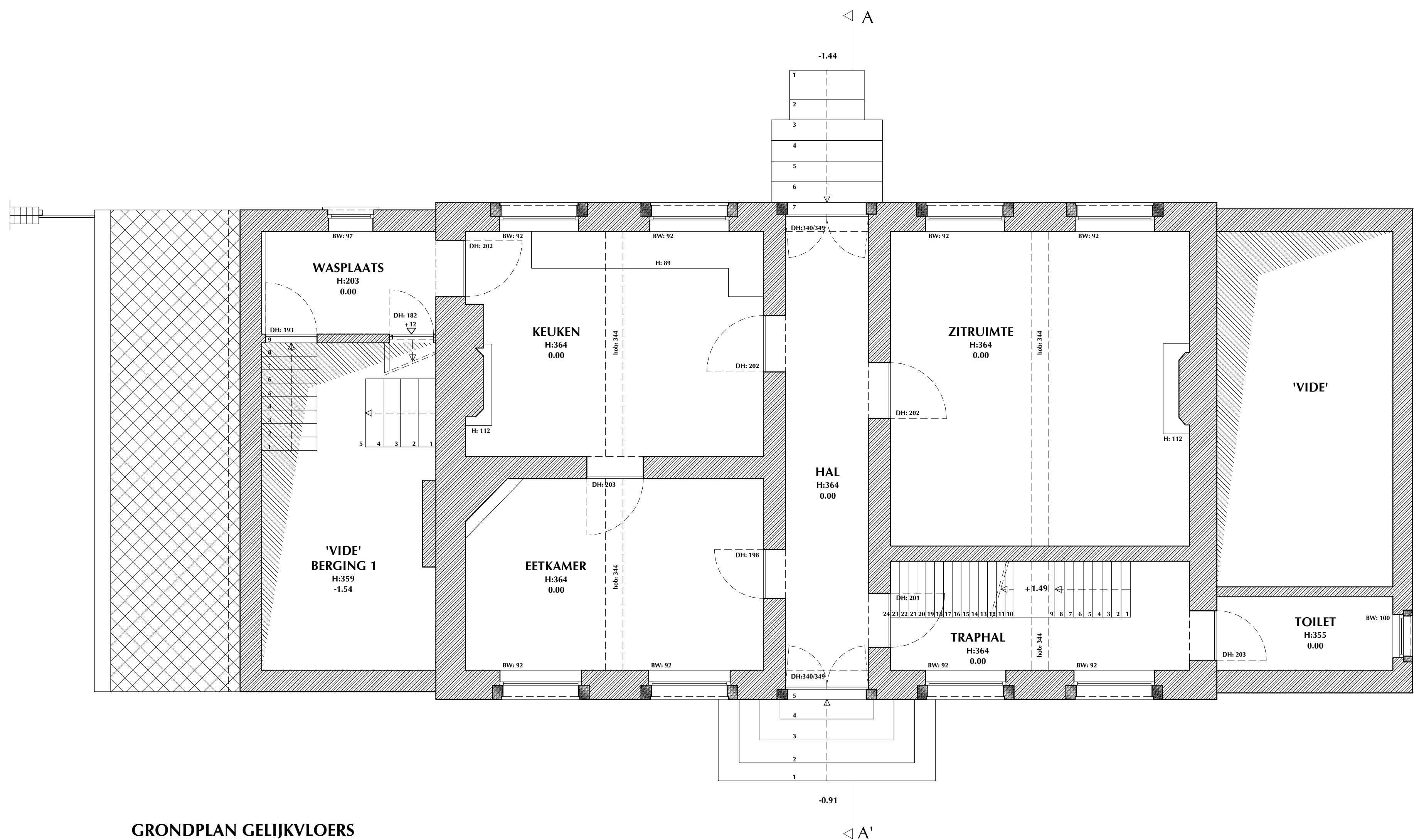
GRONDPLAN GELIJKVLOERS BESTAANDE TOESTAND schaal 1 : 50
