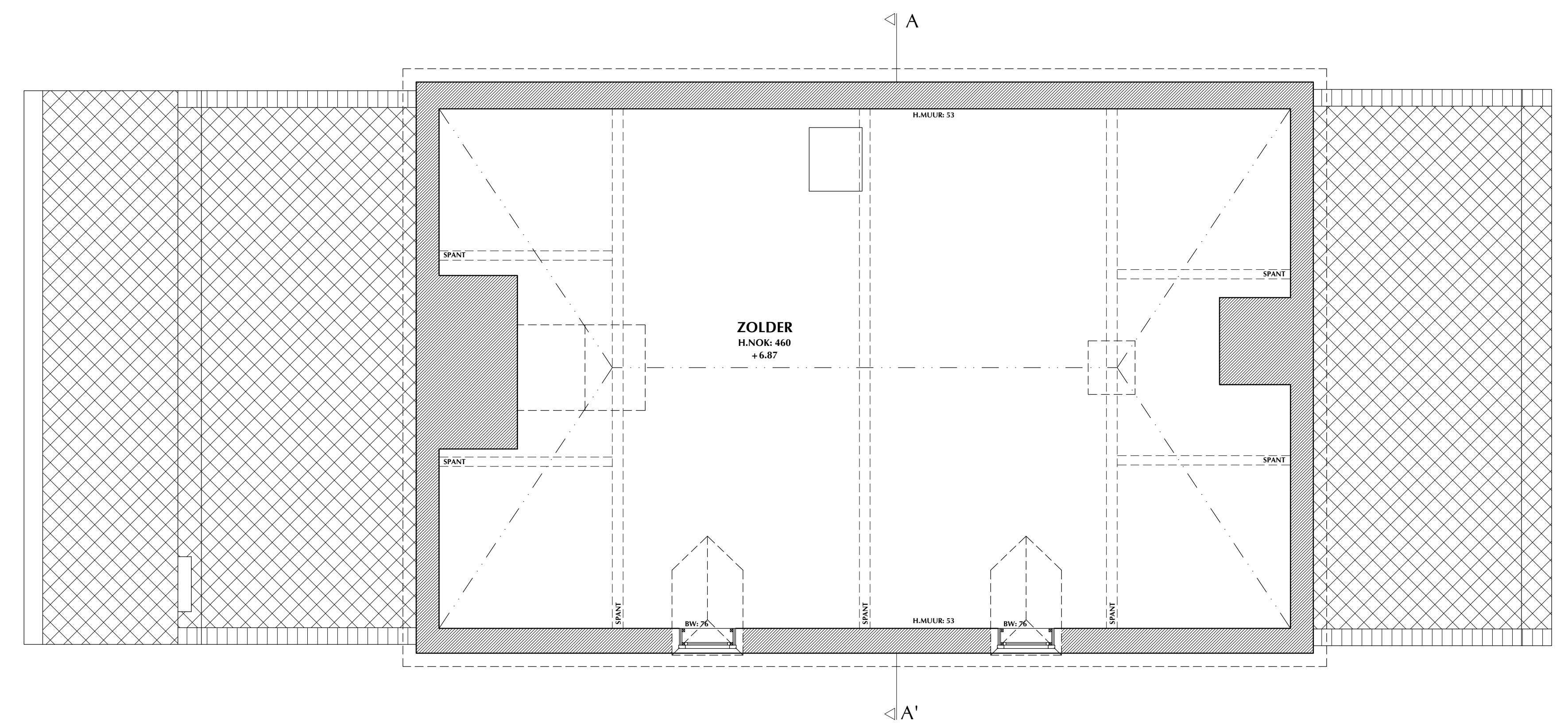
GRONDPLAN ZOLDER BESTAANDE TOESTAND schaal 1 : 50
