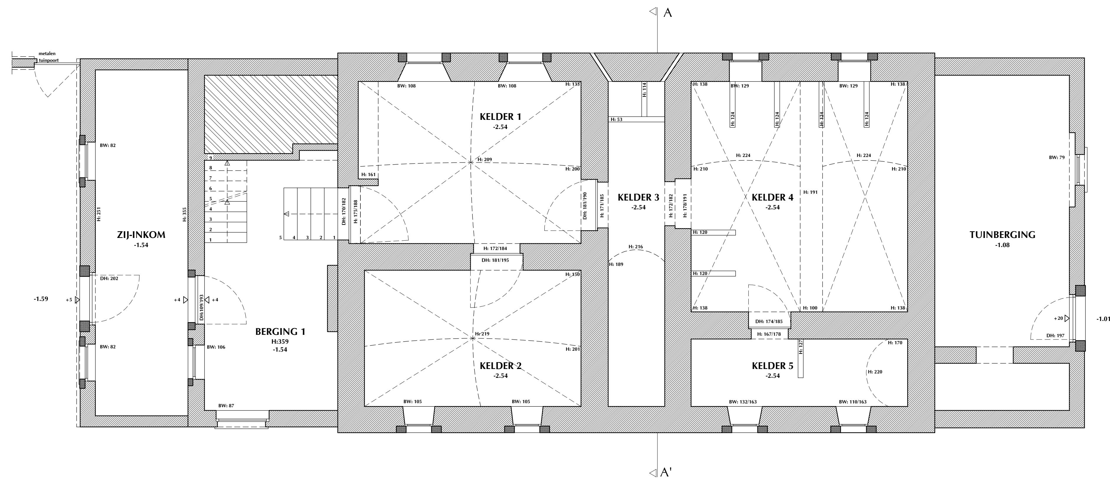
GRONDPLAN KELDER BESTAANDE TOESTAND schaal 1 : 50
