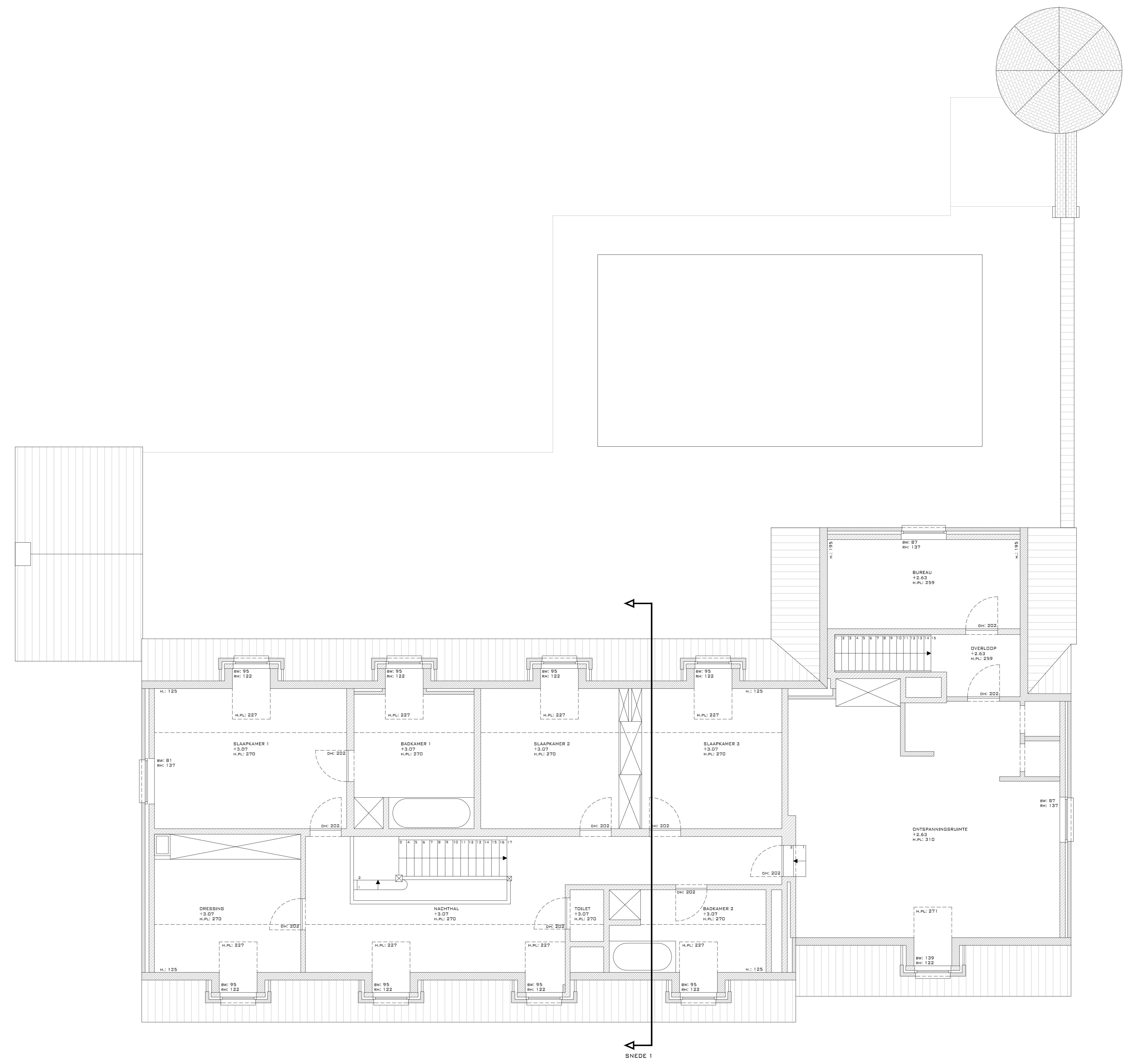
VERDIEPING
