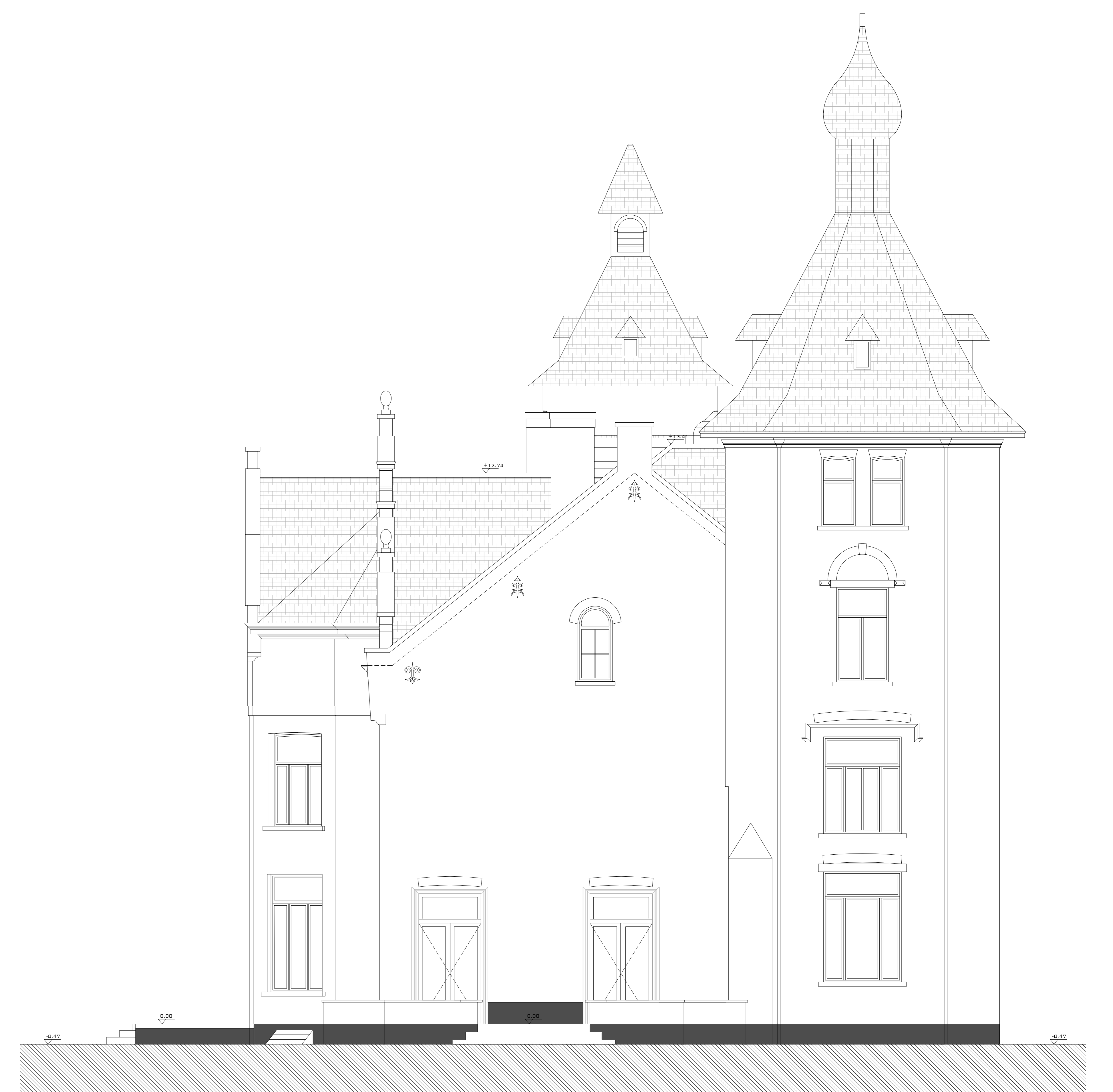
LINKER ZIJGEVEL
