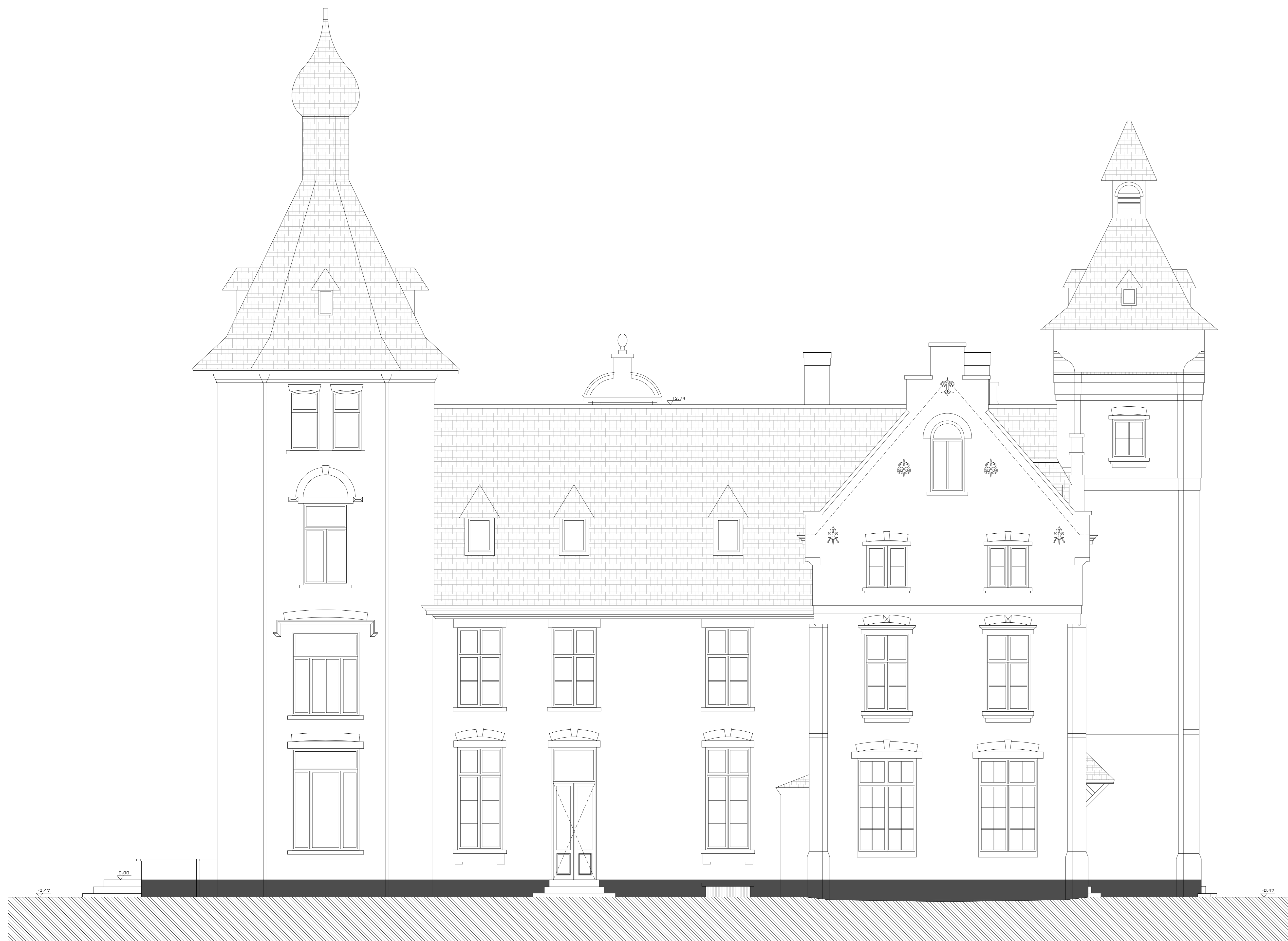
VOORGEVEL
