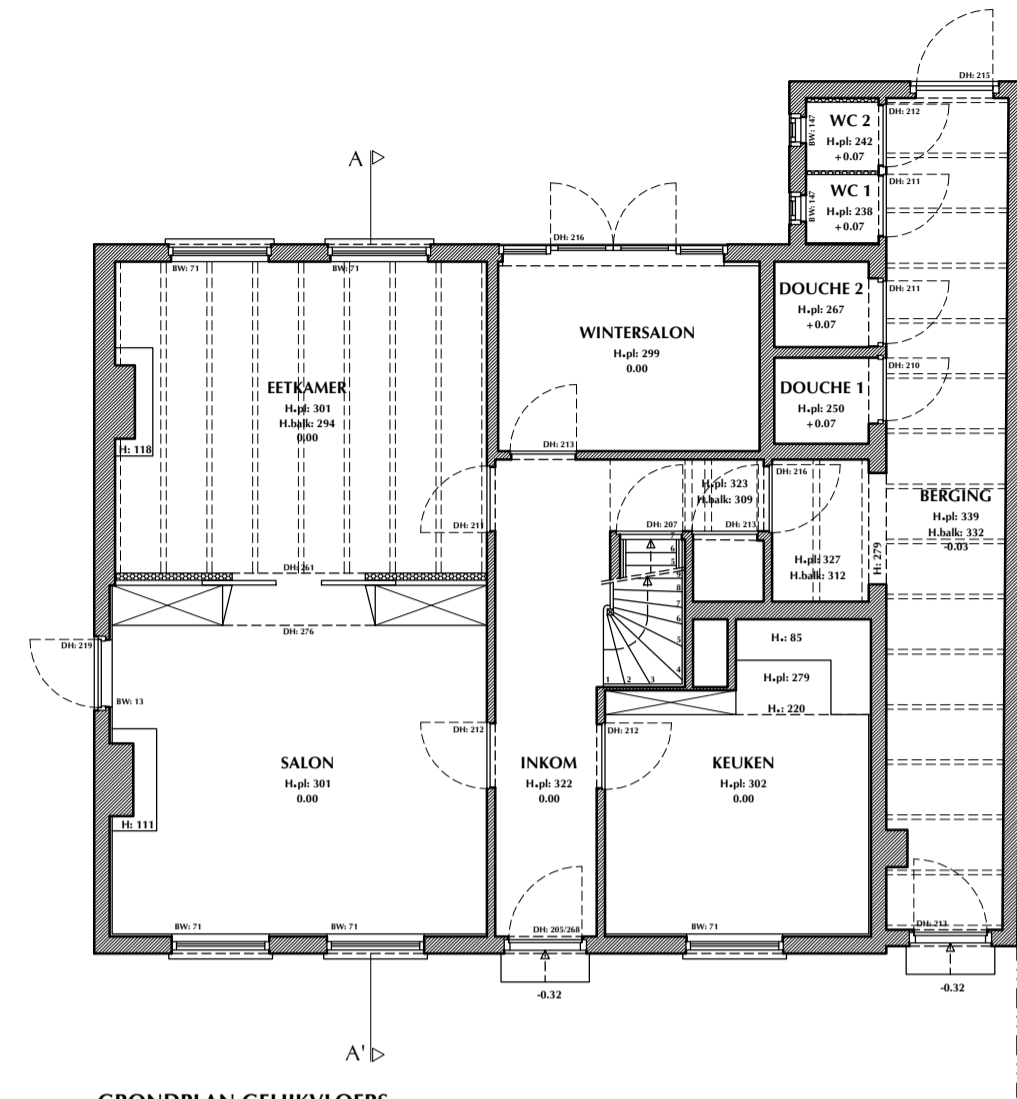
GRONDPLAN GELIJKVLOERS BESTAANDE TOESTAND schaal 1:50
