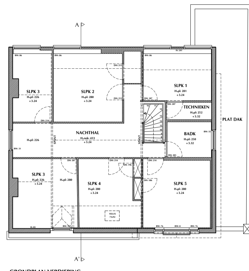
GRONDPLAN VERDIEPING BESTAANDE TOESTAND schaal 1:50
