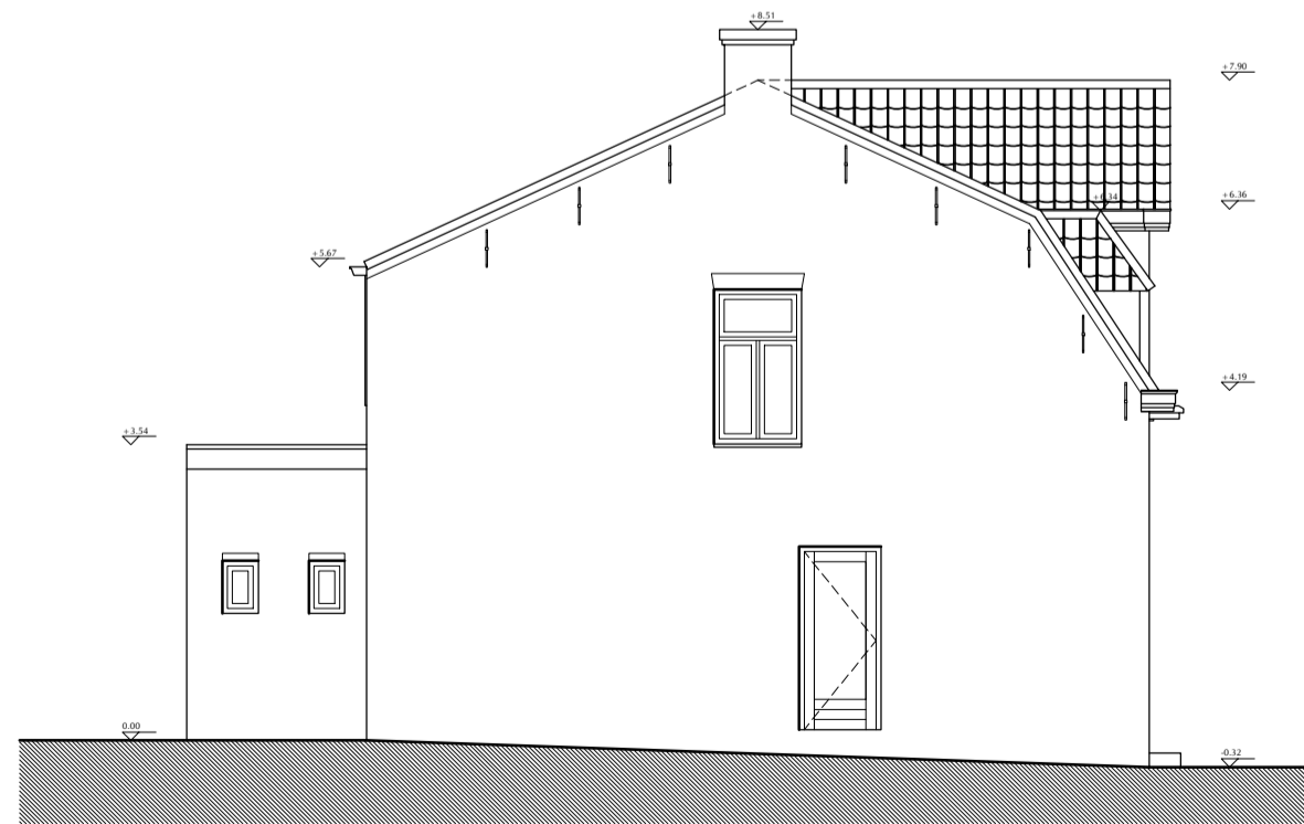
LINKER ZIJGEVEL BESTAANDE TOESTAND schaal 1:50
