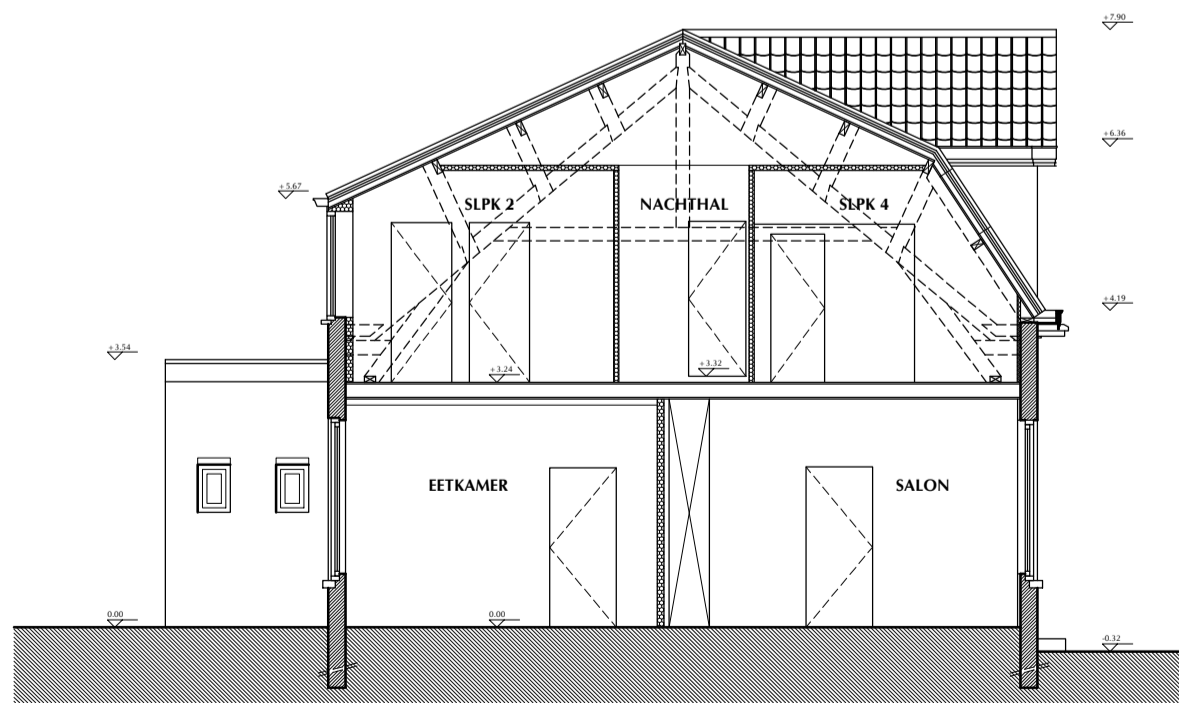
SNEDE AA' BESTAANDE TOESTAND schaal 1:50
