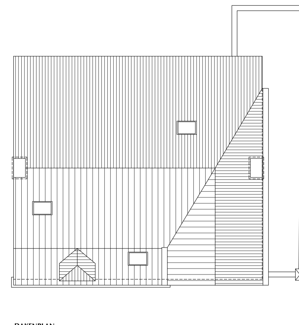
DAKENPLAN BESTAANDE TOESTAND schaal 1:50
