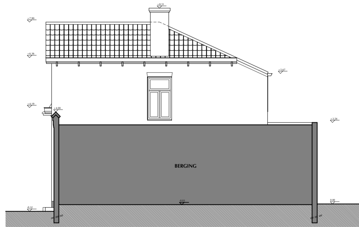
RECHTER ZIJGEVEL BESTAANDE TOESTAND schaal 1:50
